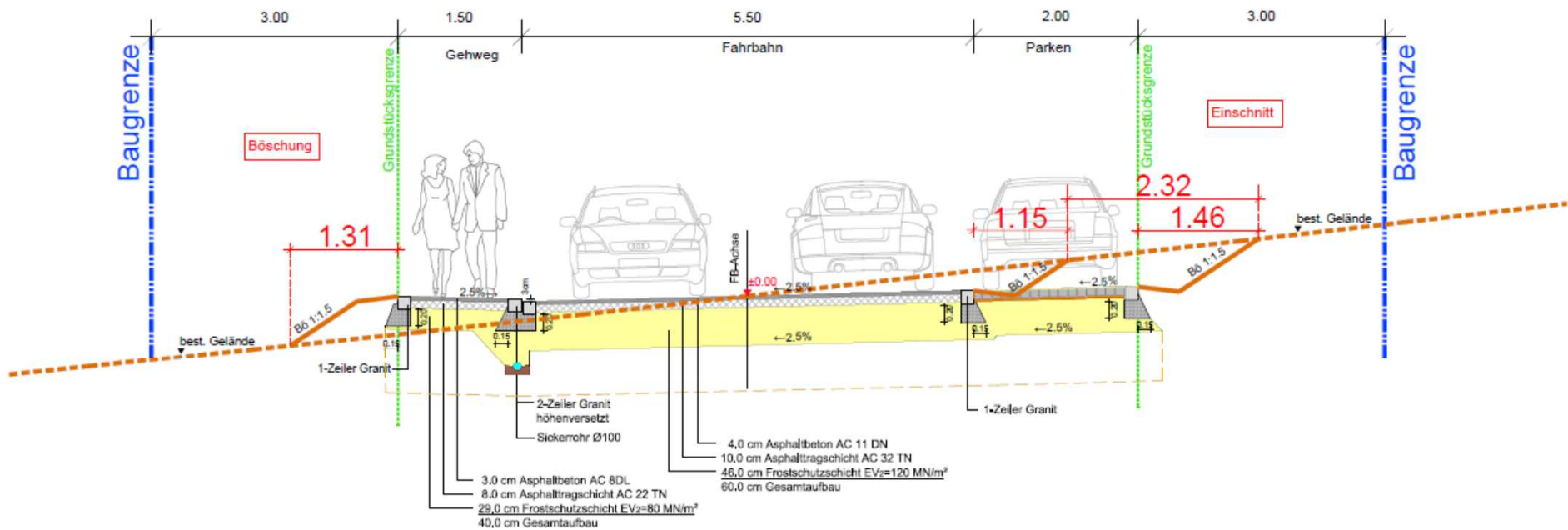
Schnitt 1 - 1 Planung Straße Geländegleich 0+120.00 Kirlesberg "B" M 1:50
